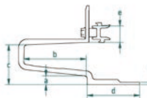
101028-020 RapidA Pro 2L tetőhorog Csom. egys.: 30
