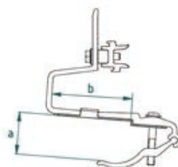
109019-025 Pro- N tetőhorog Csom. egys.: 30
