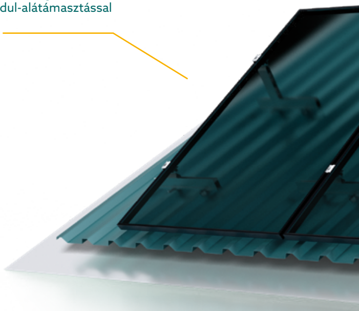
FIXZ PRO TRAPÉZLEMEZHEZ SingleFix Pro-val és Pro magasítóelem- mel / modul-alátámasztással
